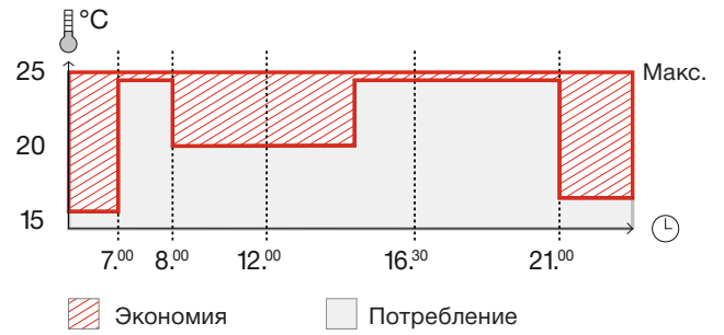
Экономия энергии за счет индивидуального управления отоплением в зависимости от времени суток
