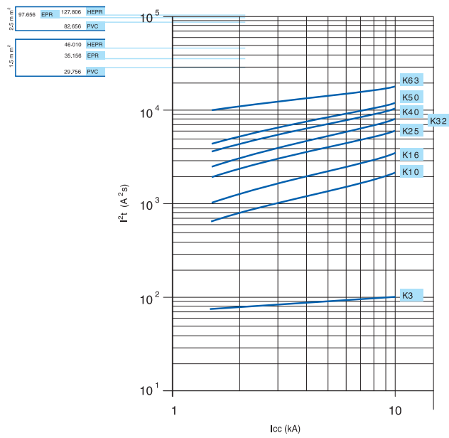
S 280 характеристики К, Z 230/400 V B
