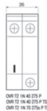
2 полюса (1P+N)
