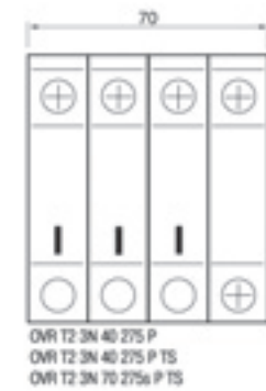
4 полюса (3P+N)
