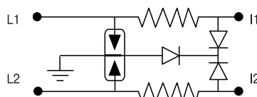
OVR TC / xx V / 200 FR при последовательном подключении
