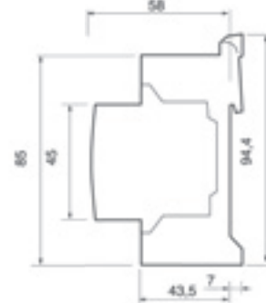
2 полюса (1P+N)
