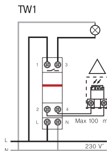
Схема подключения
