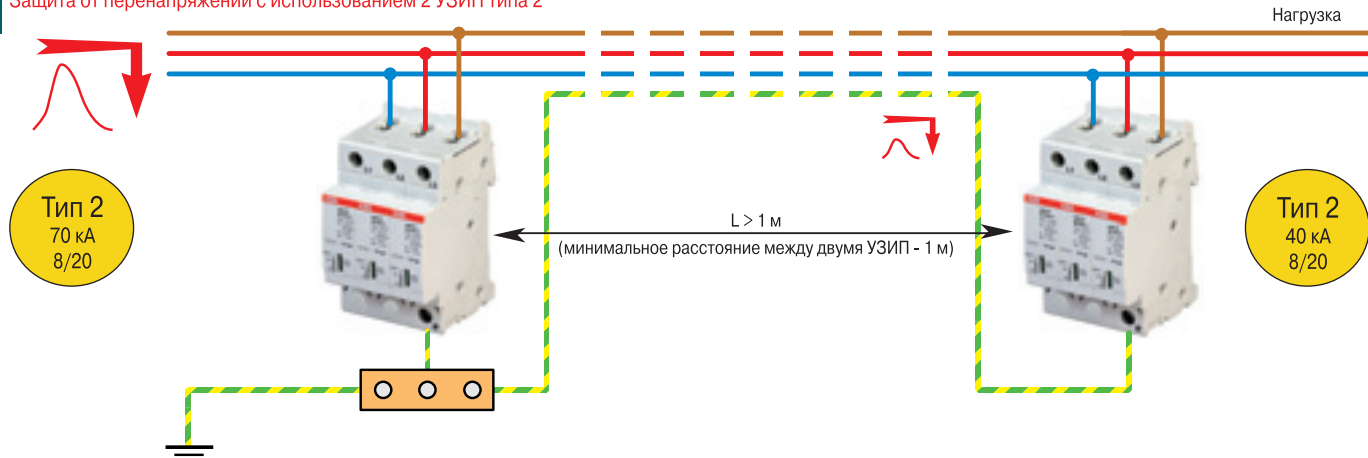
Защита от перенапряжений с использованием 2 УЗИП типа 2
