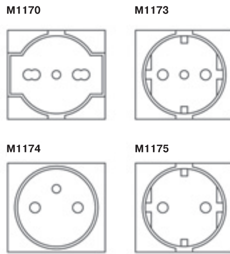
Фронтальный вид
