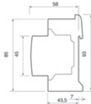
1 полюс
