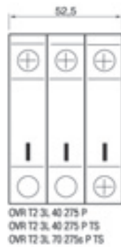
3 полюса
