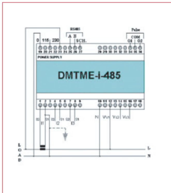
Однофазное прямое подключение
