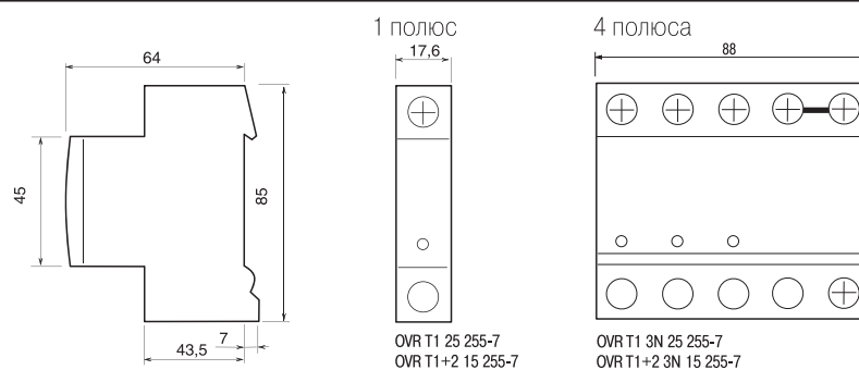
УЗИП Тип 1 и Тип 1+2 ( I_{fi} = 7 \text{ кА} )
