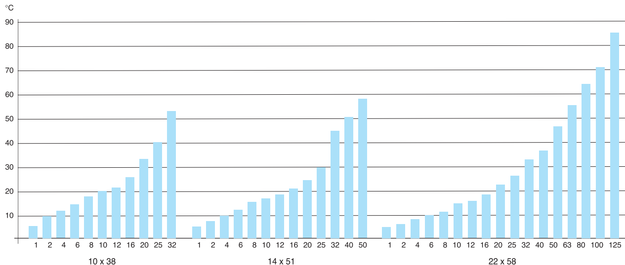
Увеличение температуры (при наилучшем контакте)
