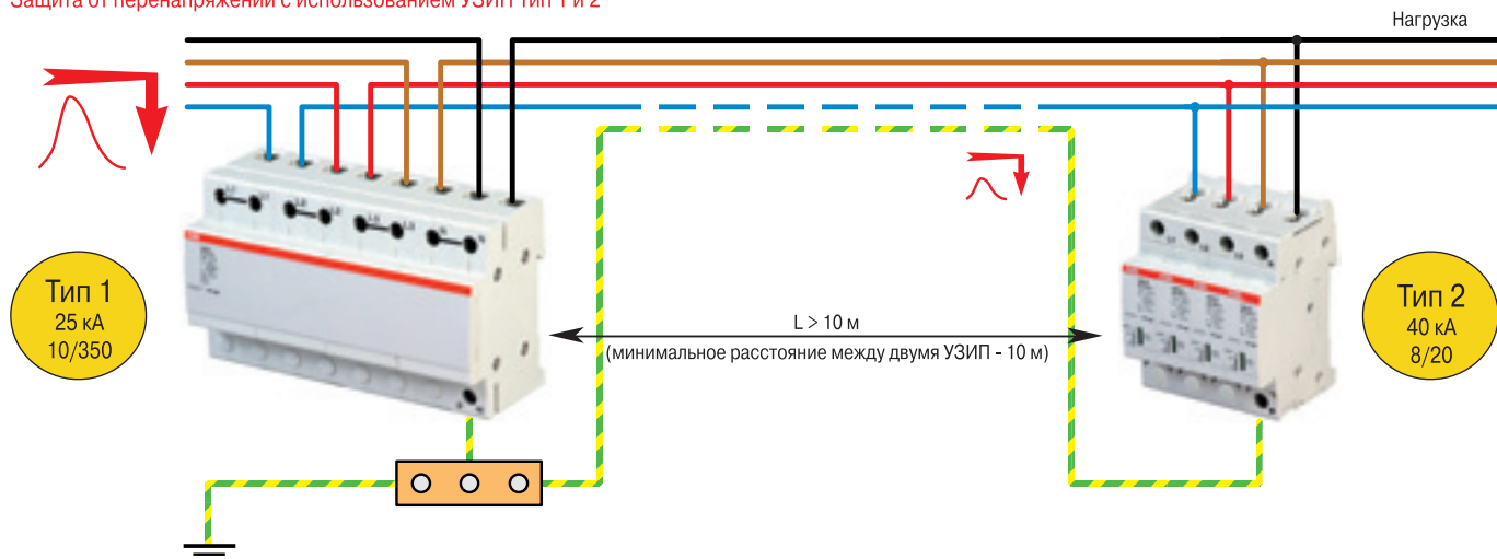
Защита от перенапряжений с использованием УЗИП Тип 1 и 2
