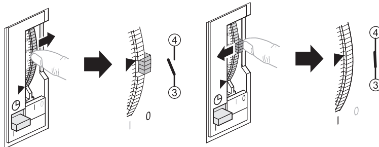
Программирование
