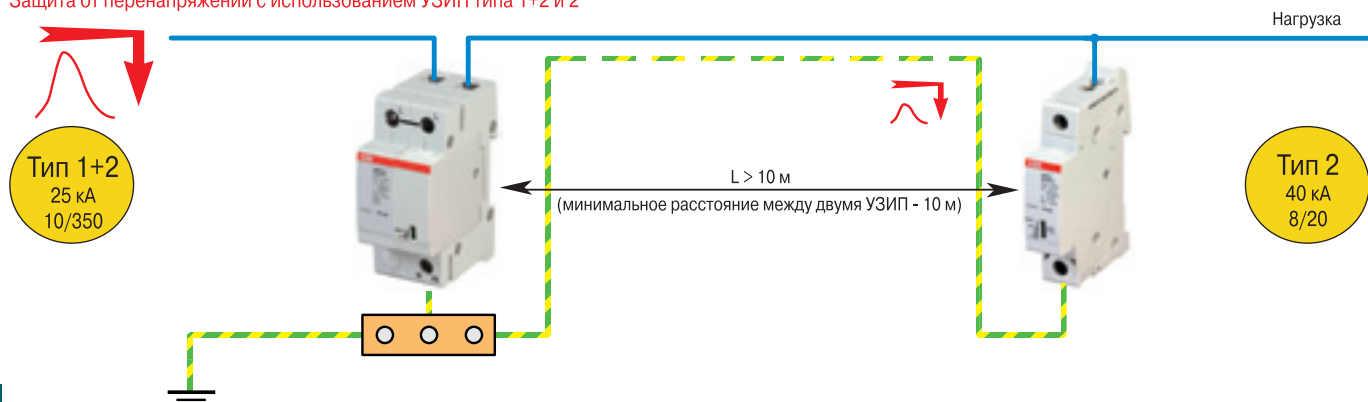
Защита от перенапряжений с использованием УЗИП типа 1+2 и 2
