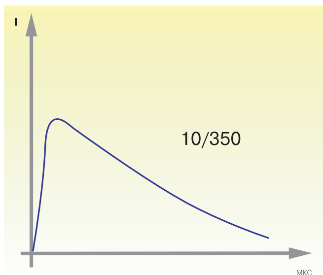
УЗИП типа 1
