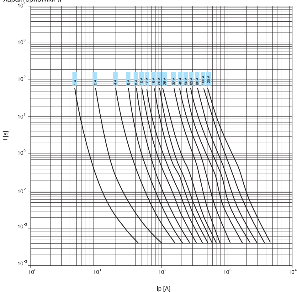
Характеристики tI
