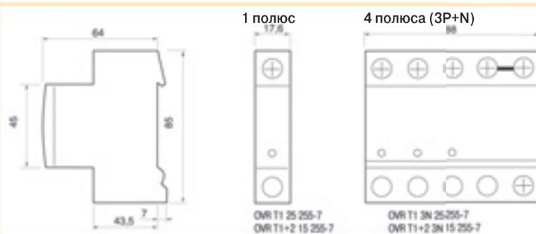
УЗИП Тип 1 и Тип 1+2 ( I_{\text{н}}=7 \text{ кА} )
