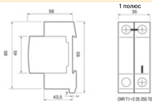
УЗИП Тип 1 и Тип 1+2 ( I_{\text{н}}=7 \text{ кА} )
