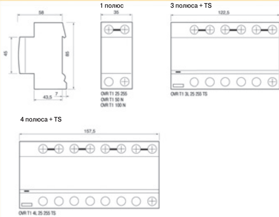
УЗИП Тип 1 ( I_{\text{н}}=50 \text{ кА} )
