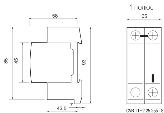
УЗИП Тип 1+2 ( I_{fi} = 15 \text{ кА} )
