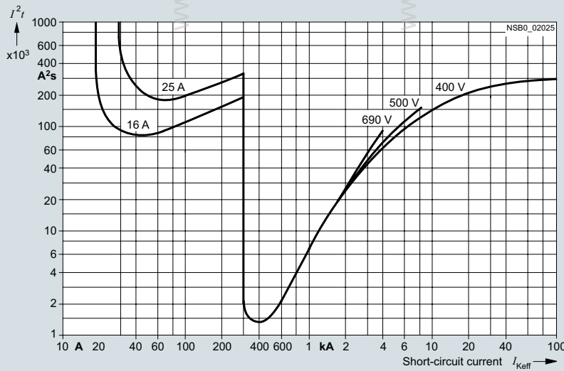
Характеристика I 2 t для 3VS1600-0MN00
