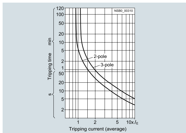
Типичные характеристики срабатывания
