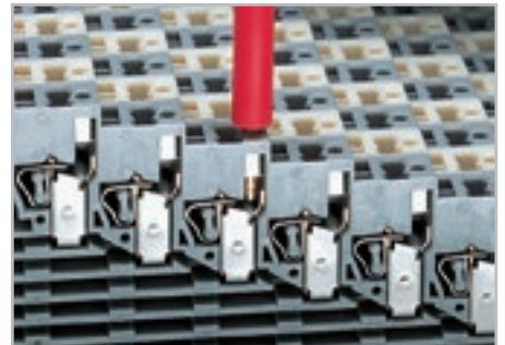
Специальный тестовый контакт для тестового штекера 2,3 мм Ø.
