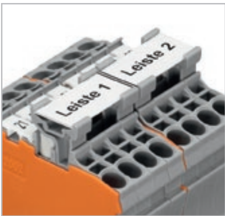
Держатели маркировочной полосы для установки в гнездах для перемычек
