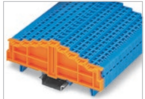
Синие клеммы для матричной коммутации пригодны для применения в условиях Ex i.
