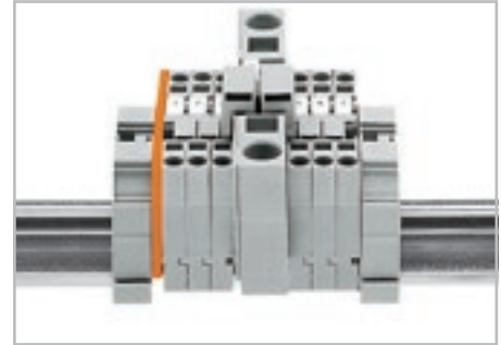
Объединение клемм от 16 мм²/AWG 6 (серия 283) до 4 мм²/AWG 12 (серия 281) для монтажа на рейку.
