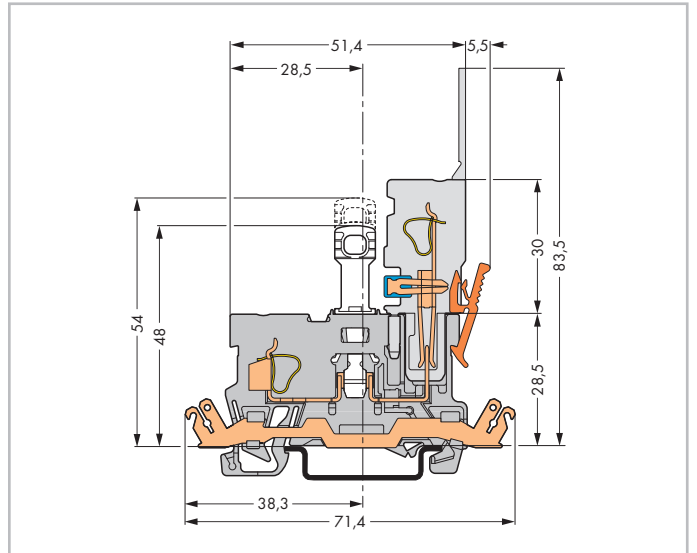
Базовая клемма с экранированным контактом и размыкателем
