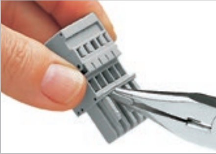
Кодировка розетки – выломайте кодировочные выступы. Не удаляйте первый и последний кодировочные выступы.
