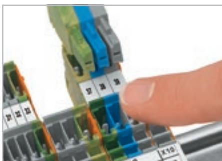
Базовые клеммы и штеккер-розетки защищены от случайного контакта.
