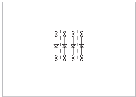
Поляризованная диодная схема, общий катод
