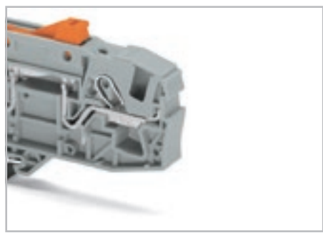
Блокировочная крышка для неиспользуемых зажимов клемм TOPJOB® S серии 2006.
