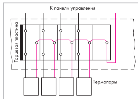
Электропитание со стороны исполнительного устройства
