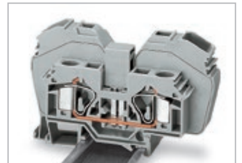
Клеммы серии 285 могут объединяться с клеммами серии 283: 285-635 или 285-634 с 283-601 или 283-604
