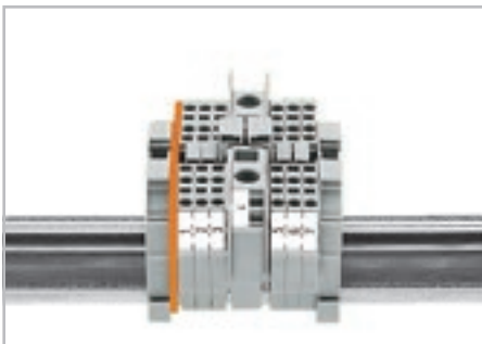
Объединение клемм от 6 мм²/AWG 10 (серия 282) до 1,5 мм²/AWG 16 (серия 279) для монтажа на рейку.
