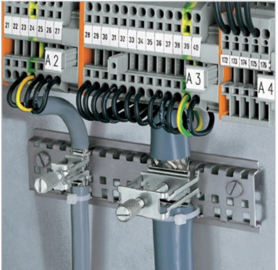
Держатель с 2 контактными ножками*, длина 125 мм, шина параллельна рейке Код 790-115 * для всех размеров зажимных скоб экрана
