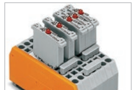
Базовые клеммы для датчиков перемычки «гребень через один» 3-кан., гребешковая перемычка
