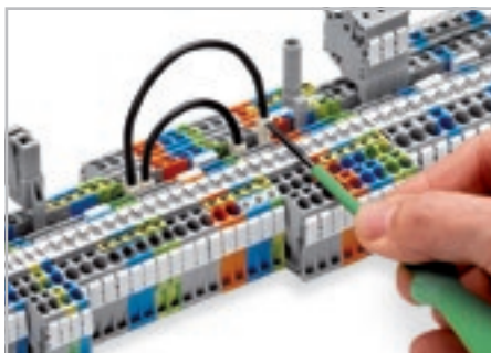
Установите удлинительную перемычку до упора. Поднимите перемычку с помощью рабочего инструмента для повторного монтажа.
