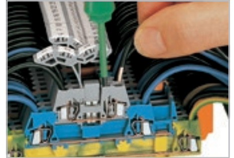
Зажим проводника
