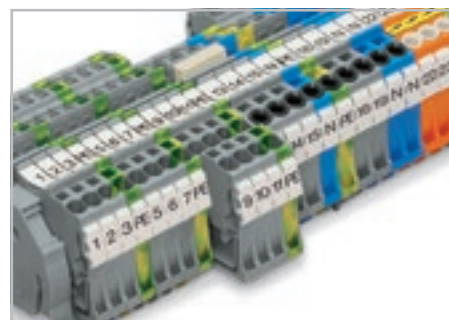
Маркировочная полоса для центральной маркировки
