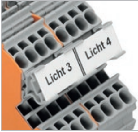
Держатели маркировочной полосы для установки в поперечные маркировочные разъемы
