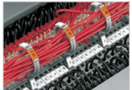
2 x групповая маркировка сверху 1 x маркировка клеммы внизу
