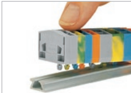
Клеммная колодка с опорными ножками, монтируются на специальную алюминиевую рейку.
