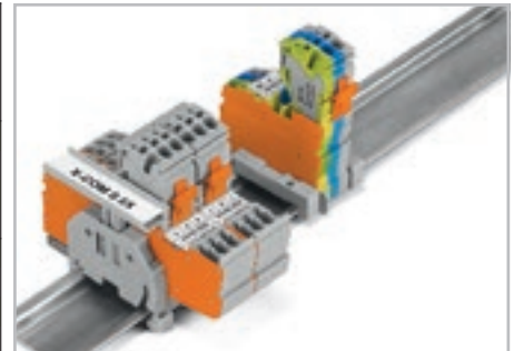
Групповая маркировка с регулируемым по высоте держателем групповой маркировки (2009-163)
