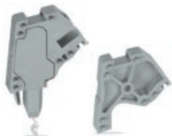
Модуль тестового штекера TOPJOB® S типа L состоит из: модули тестовых штекеров L и разделительные модули
