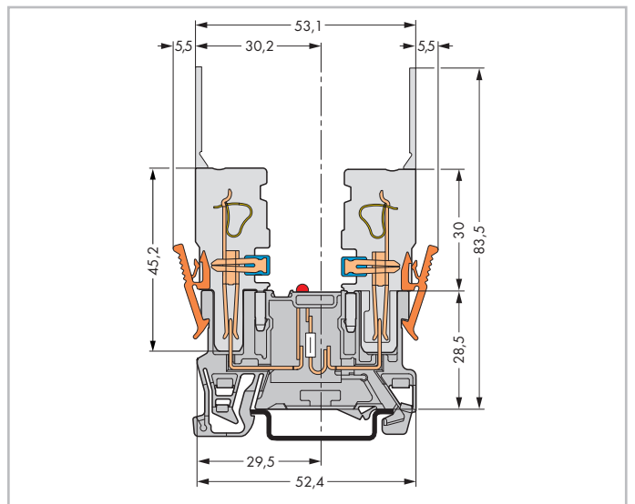
Светодиодная несущая клемма
