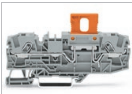
Базовая клемма с размыкателем в рабочем положении.
