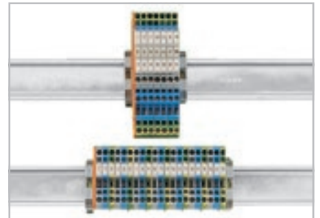
Сохраните 67% пространства рельса, используя трехуровневые клеммы.
