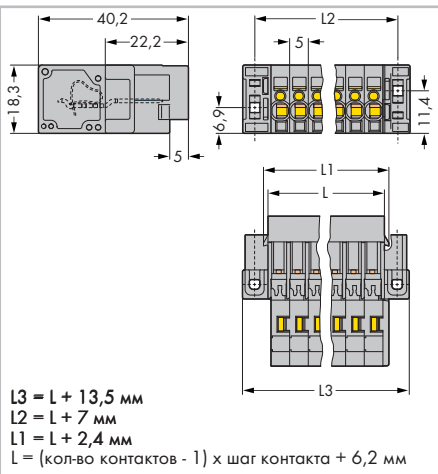
Вилка с зажимом CAGE CLAMP® с системой быстрой маркировки mini-WSB
