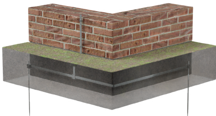
Кольцевое заземление
