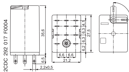
CR-M с 3 переключающими контактами
