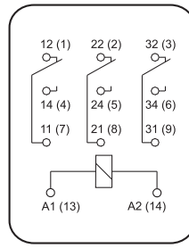
CR-M с 3 переключающими контактами
