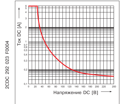
CR-M с 4 переключающими контактами
