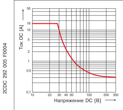
CR-P с 1 переключающим контактом
