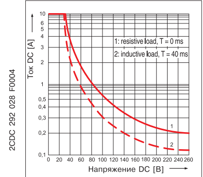
CR-U с 2 и 3 переключающими контактами
