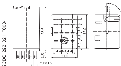
CR-M с 4 переключающими контактами
