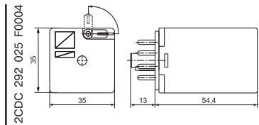
CR-U с 2 переключающими контактами
