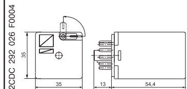
CR-U с 3 переключающими контактами
