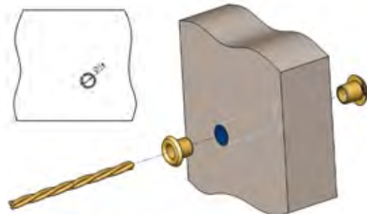
Aplicación del tapón pasamuros Use of the wall-passing cap Application du bouchon passe-murs
