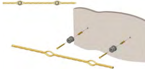
Instalación de cable trenzado con aisladores Installation of intertwined cable with insulators Installation de câble torsadé avec isolateurs
