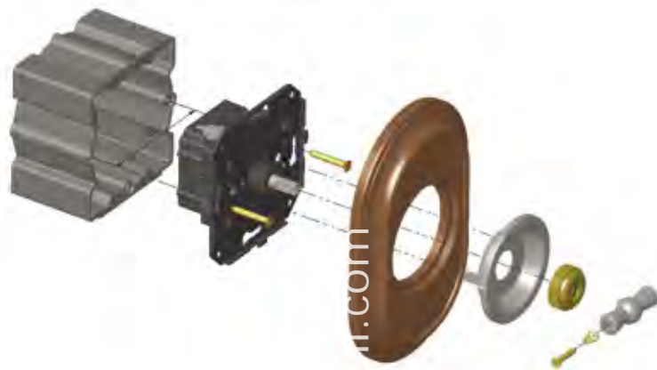
A Montaje de mecanismo Venezia Assembling of Venezia mechanism Montage du mécanisme Venezia
