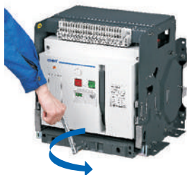
Рис. 5. Выкатывание выключателя
