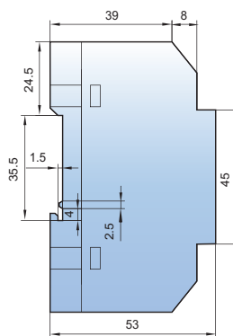
Размеры присоединяемых шин
