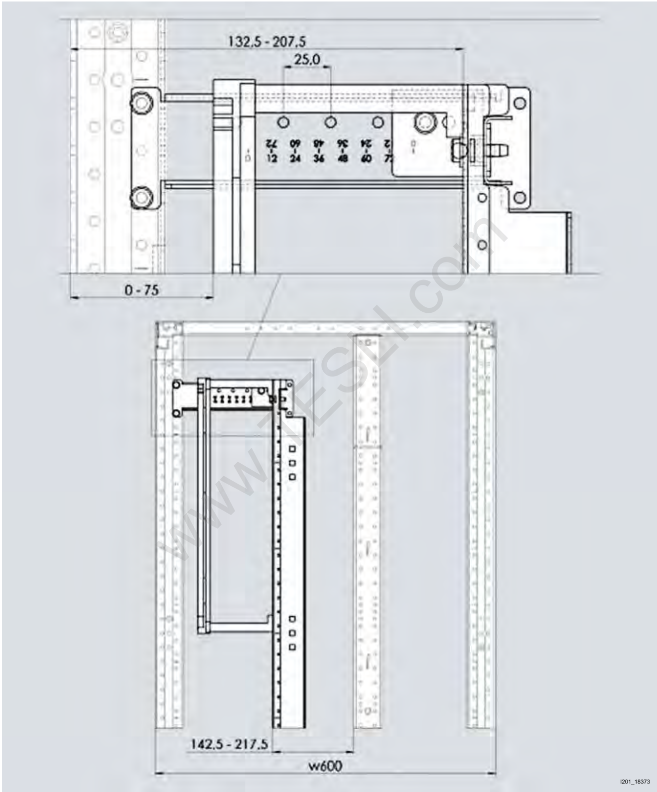
Каркас глубиной 400 мм, глубина установки спереди
